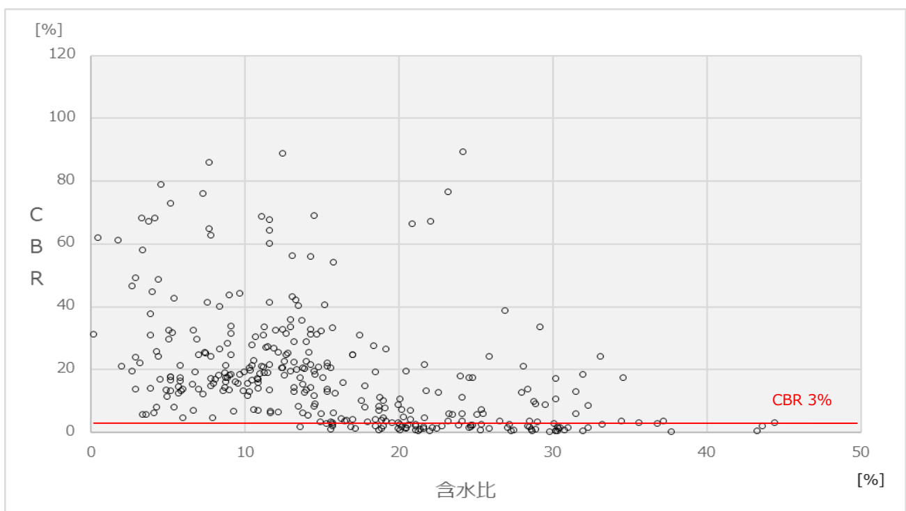
図-8 含水比とCBRの関係(砂質土)
