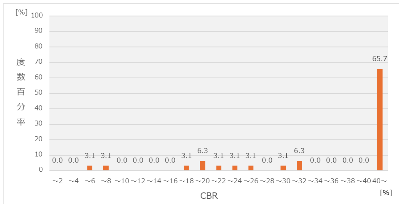
図－5 CBRの分布(れき質土)
