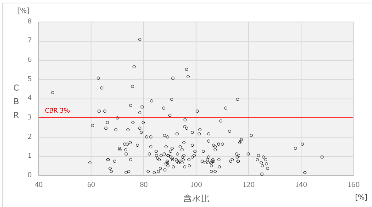
図－１２ 含水比とC B R の関係(火山灰質細粒度)
