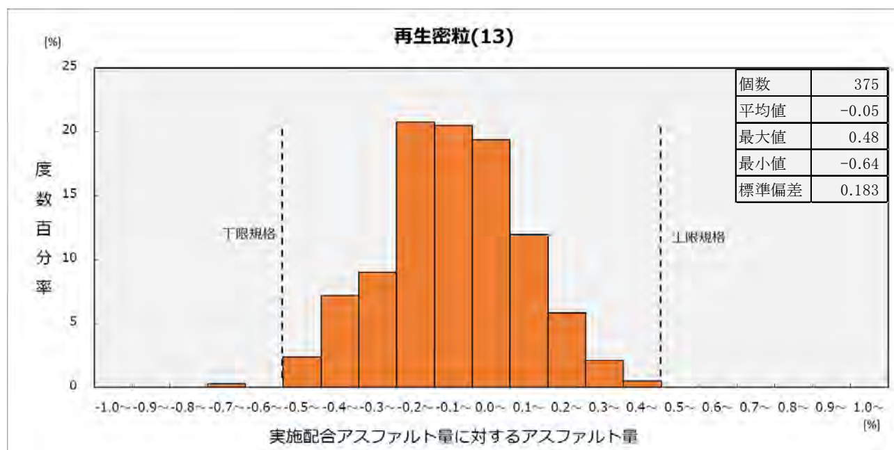
図3－（2）アスファルト量ヒストグラム
