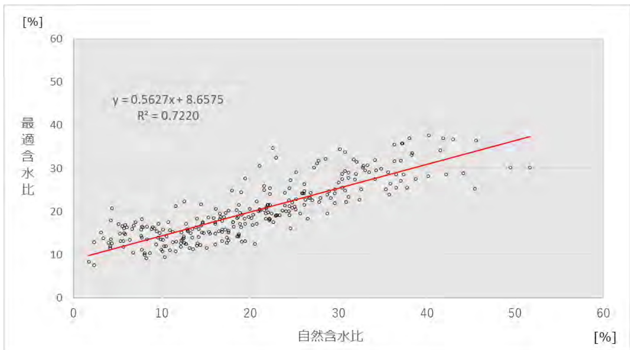
図－１ 自然含水比と最適含水比の関係（砂質土）
