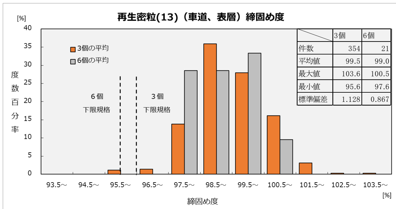
図ー 6 (2) 締固め度ヒストグラム
