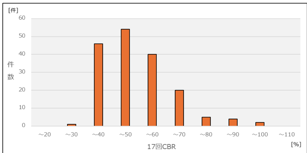
図-7 17回CBRの分布(RB-40)
