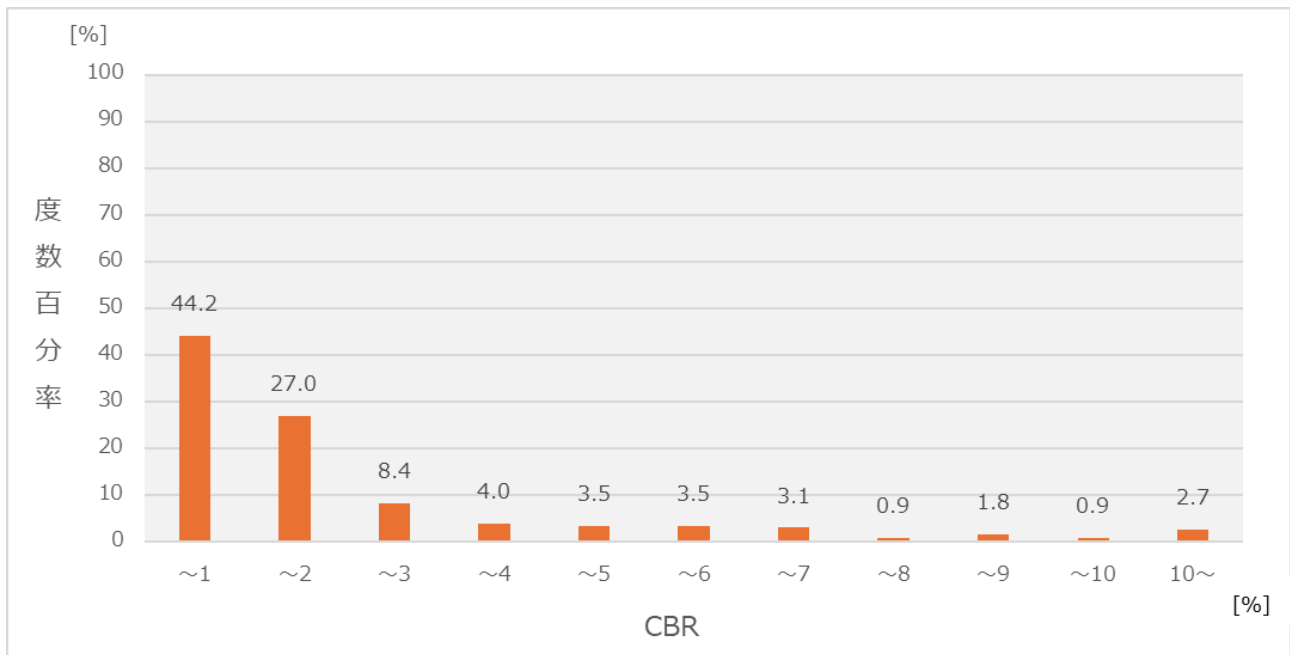
図－9 CBRの分布(粘性土)
