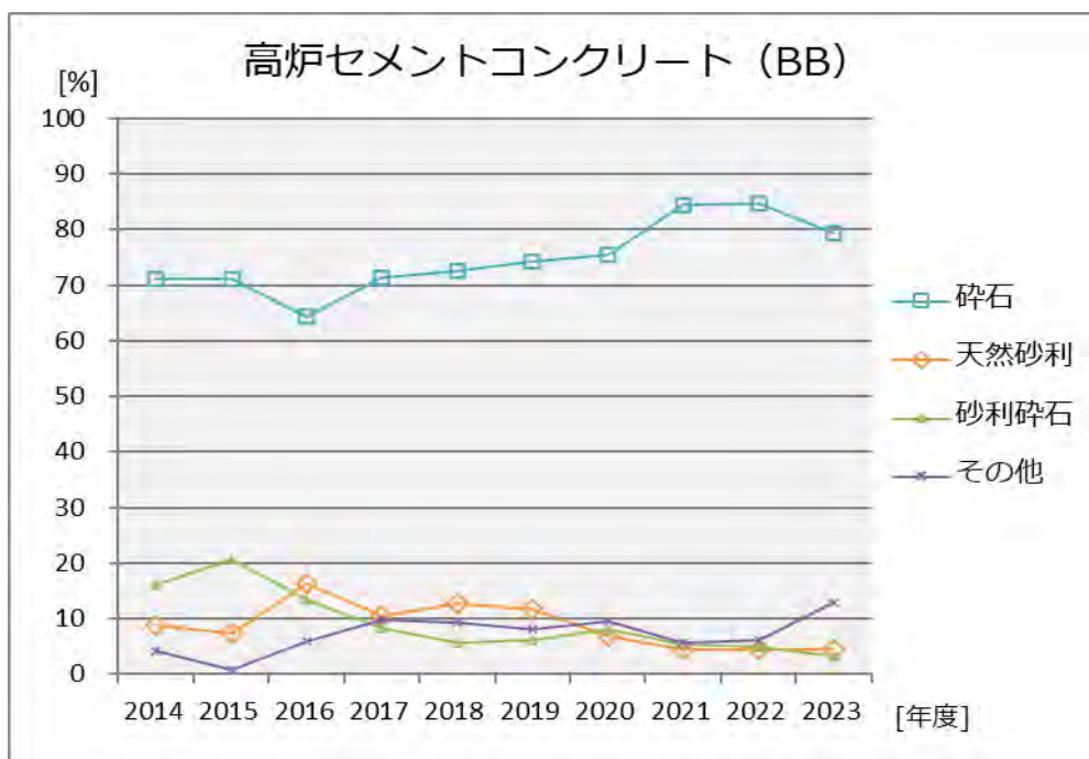
図 2 - 1 (3) 年度別粗骨材使用割合
