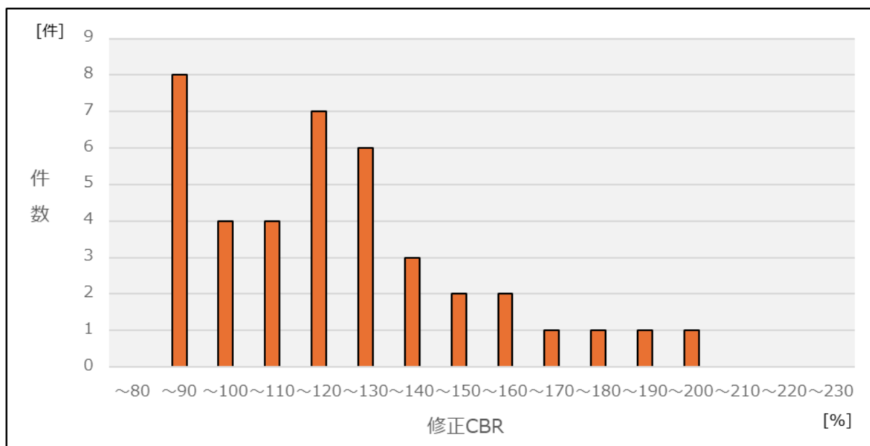
図－3 修正CBRの分布(M－30)
