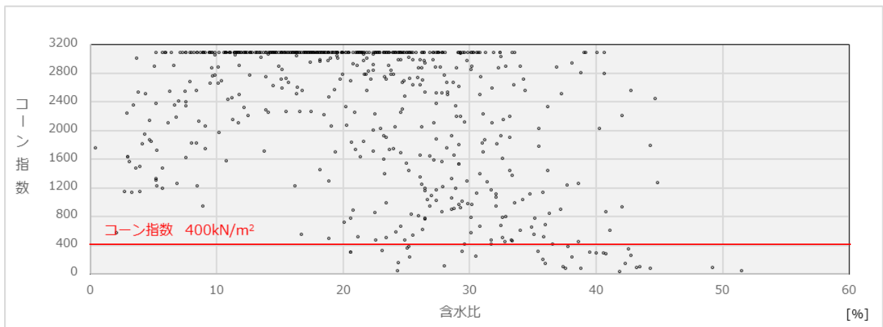
図－１９ コーン指数と含水比の関係(砂質土)
