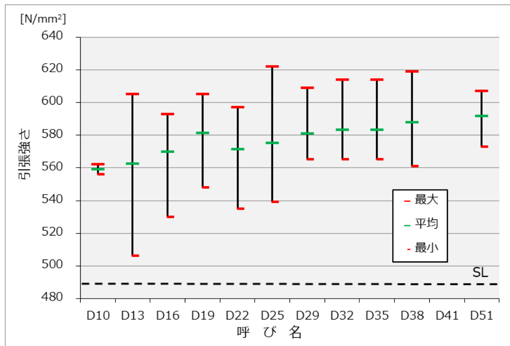
図－6 引張強さの範囲 (SD345)
