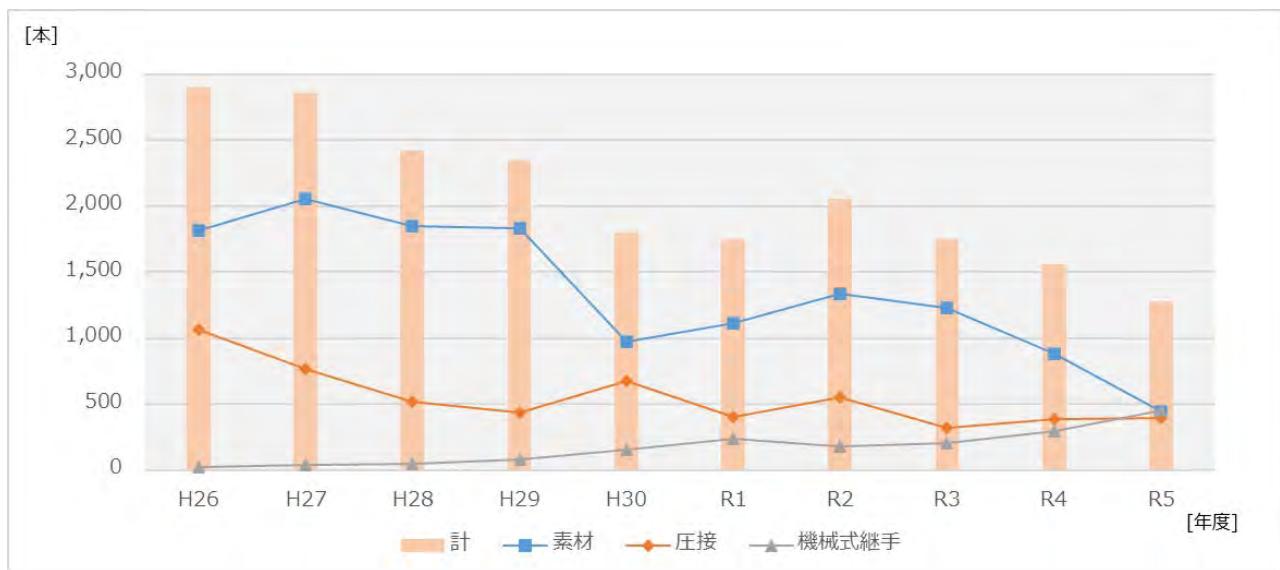
図－10 各種鉄筋コンクリート用棒鋼の依頼推移
