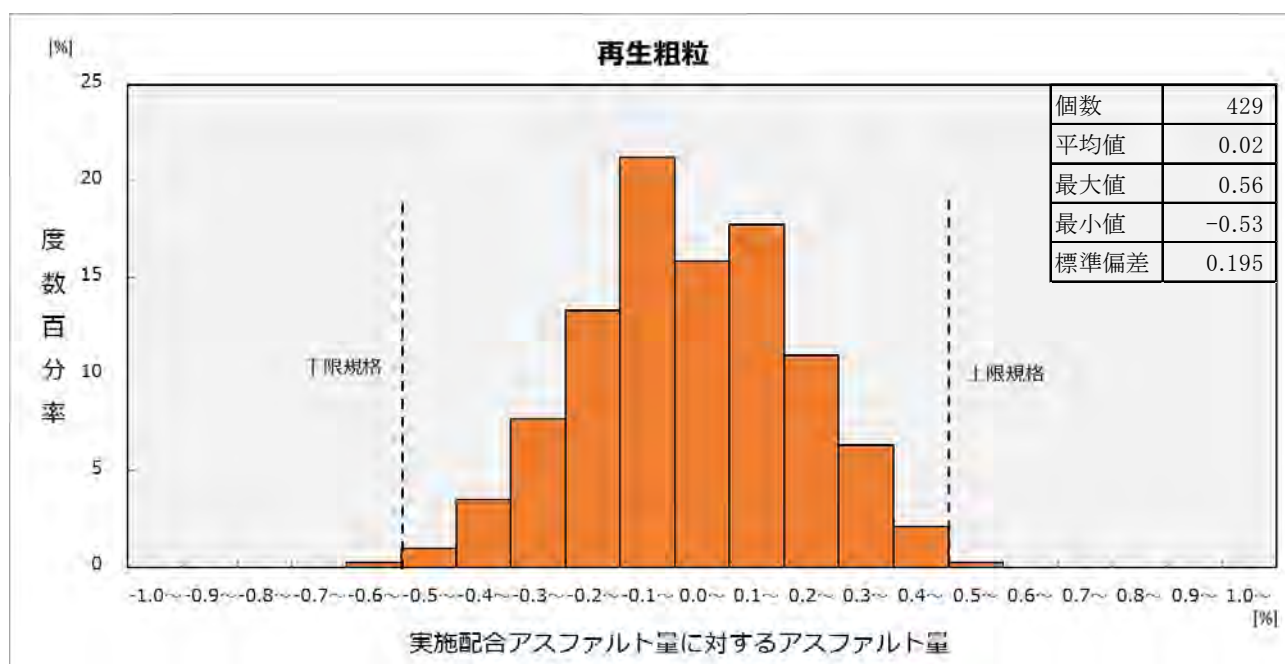
図 3 - (3) アスファルト量ヒストグラム
