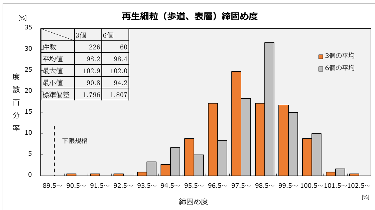
図一6（4） 締固め度ヒストグラム
