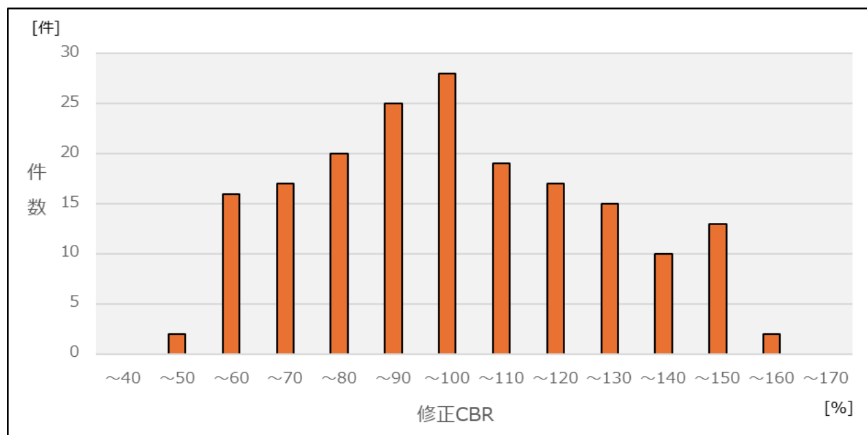
図-6 修正CBRの分布(RC-40)
