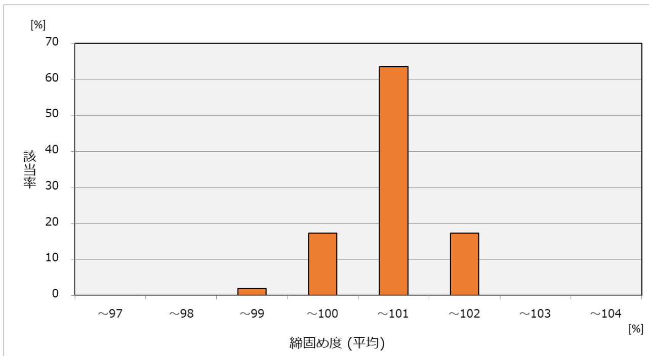
図－ 9 （ 1 ） 締固め度 再生改質Ⅱ型密粒（ 2 0 ）
