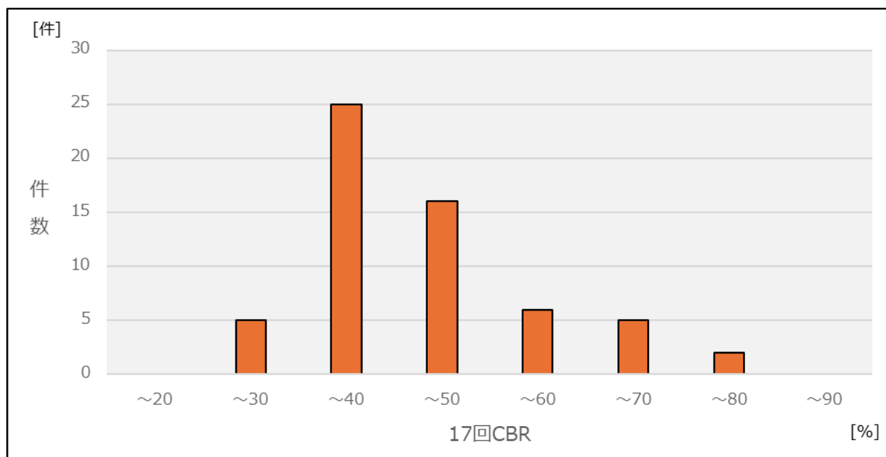
図－5 17 回 C B R の分布 (路床用碎石)
