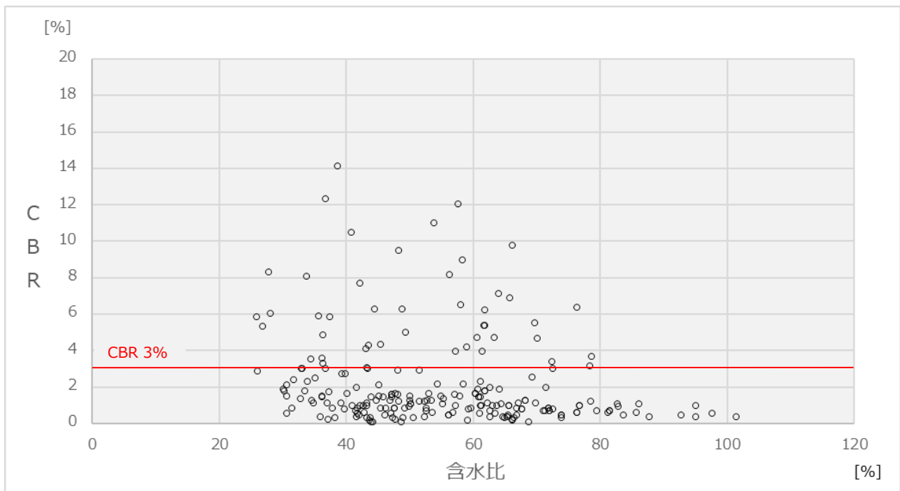
図－10 含水比とCBRの関係(粘性土)
