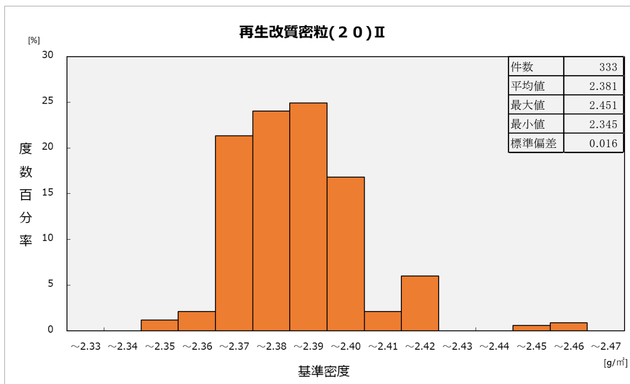
図ー 5 （ 5 ） 基準密度ヒストグラム
