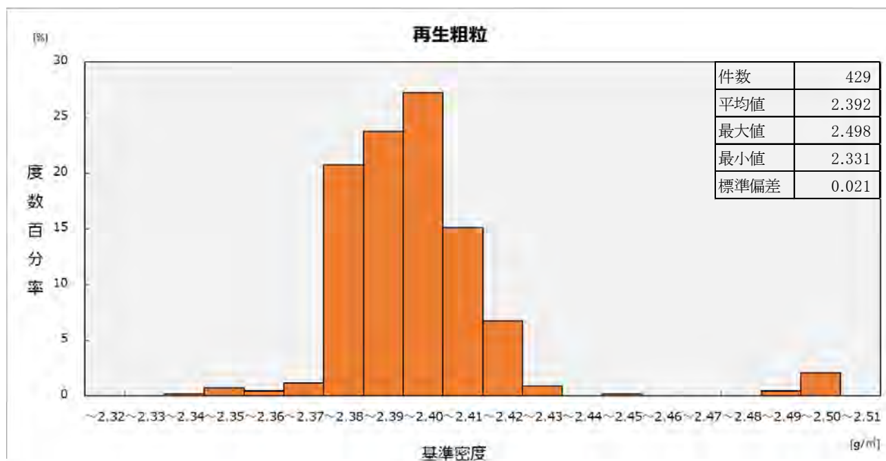
図ー 5 （ 3 ） 基準密度ヒストグラム
