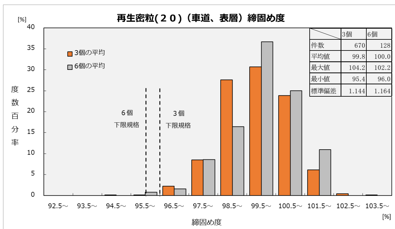
図－6（１） 締固め度ヒストグラム
