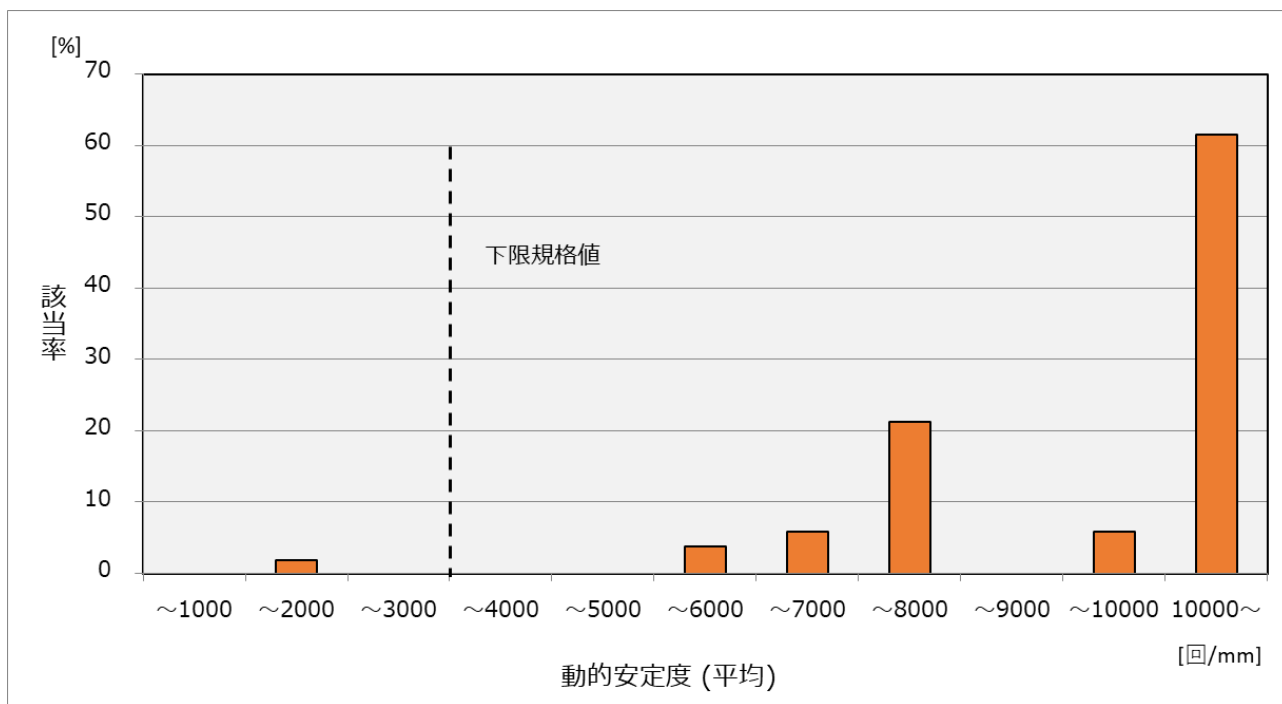
図－ 9 （ 2 ） 動的安定度 再生改質Ⅱ型密粒（ 2 0 ）
