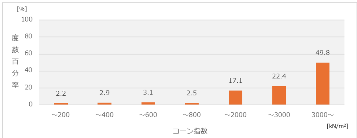
図－１６ 砂質土
