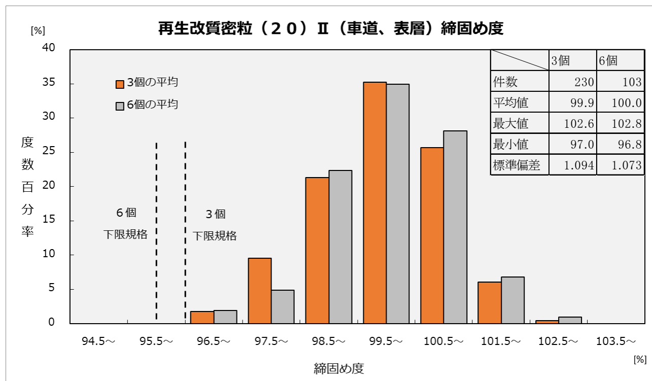
図一6（5） 締固め度ヒストグラム
