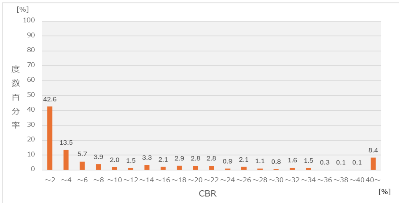
図－１３ CBRの分布
