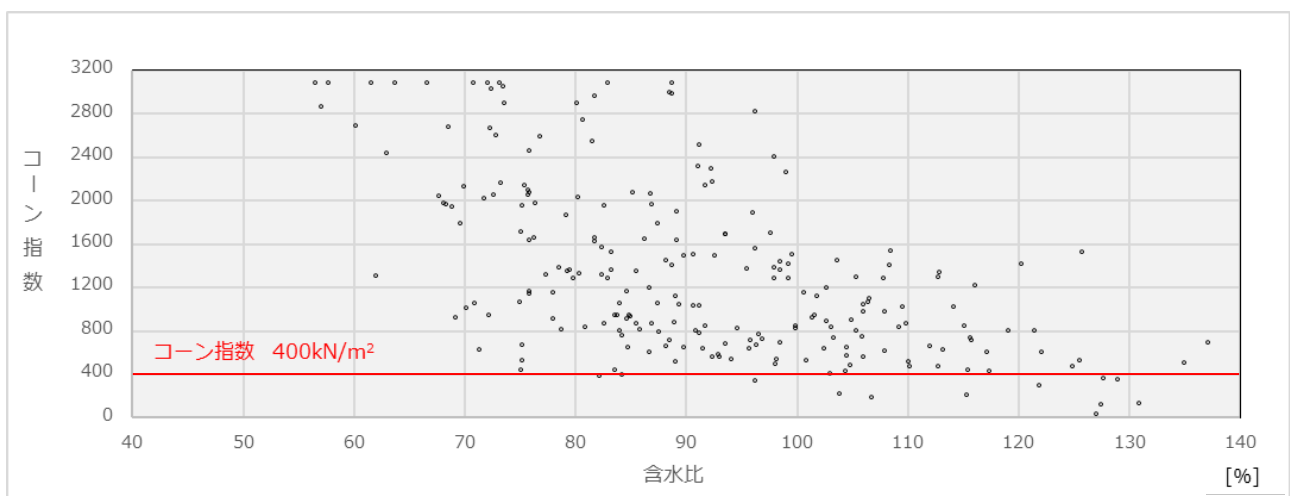
図－２１ コーン指数と含水比の関係(火山灰質細粒土)
