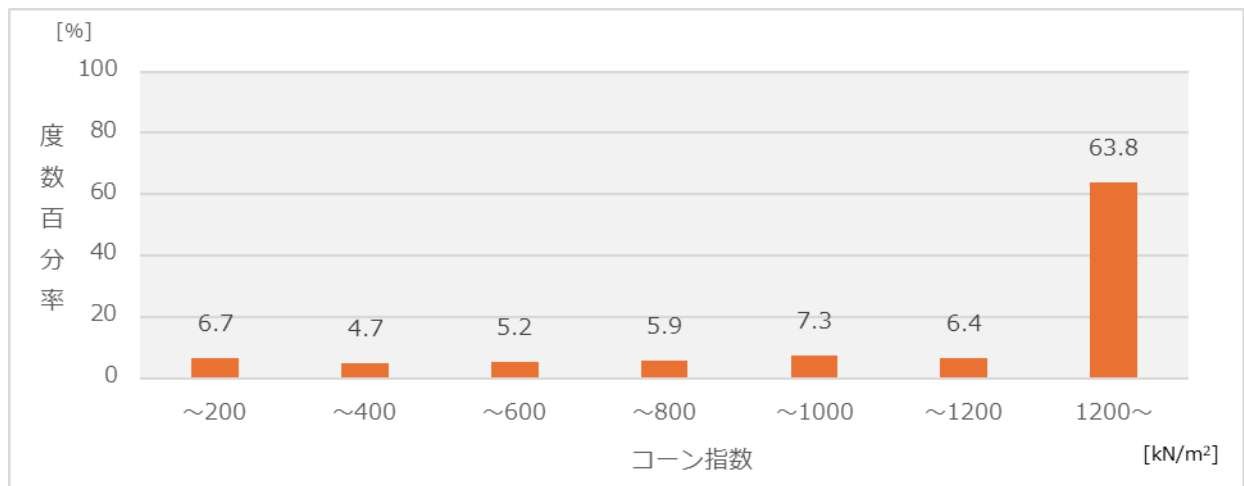
図－１７ 粘性土
