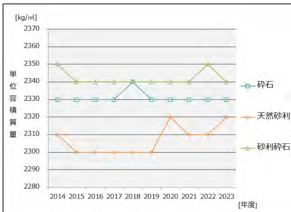
図 2 - 2 年度別の粗骨材別によるコンクリートの見掛け密度 ( \text{kg}/\text{m}^3 ) の平均値
