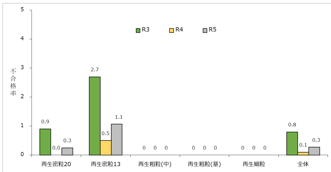
図－7 年度別締固め度不合格率
