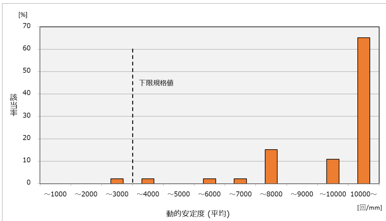
図－ 9 （ 4 ） 動的安定度 再生改質Ⅱ型粗粒
