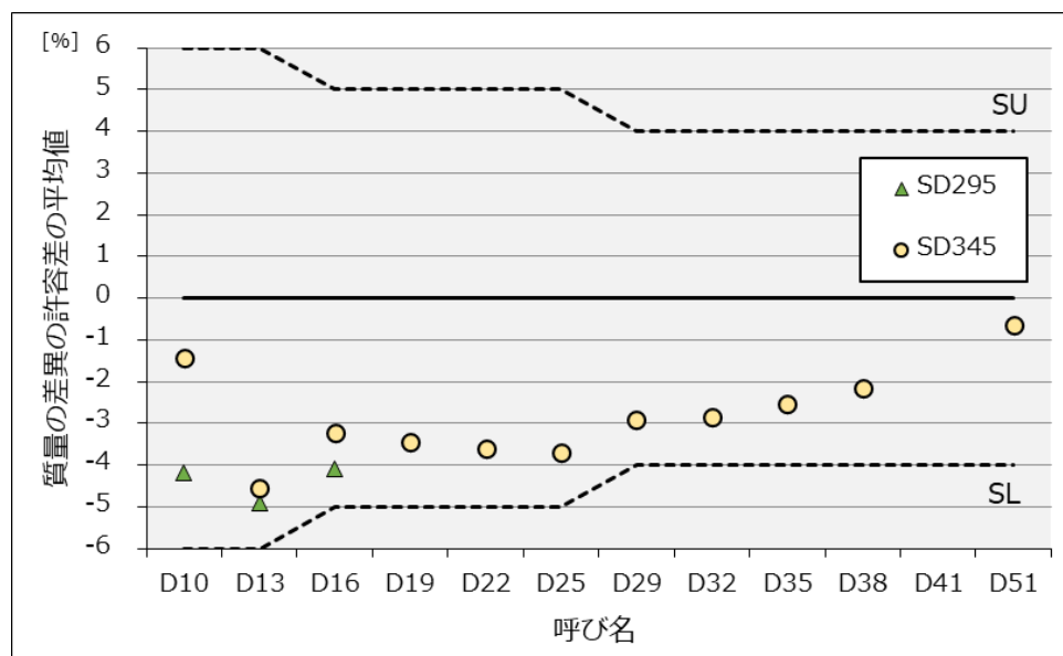
図－4 質量差異の許容差平均値
