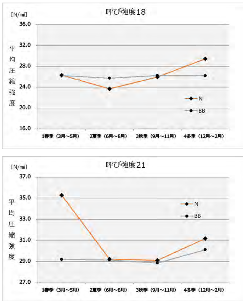
図1-2(1) 呼び強度18・21(標準養生)
