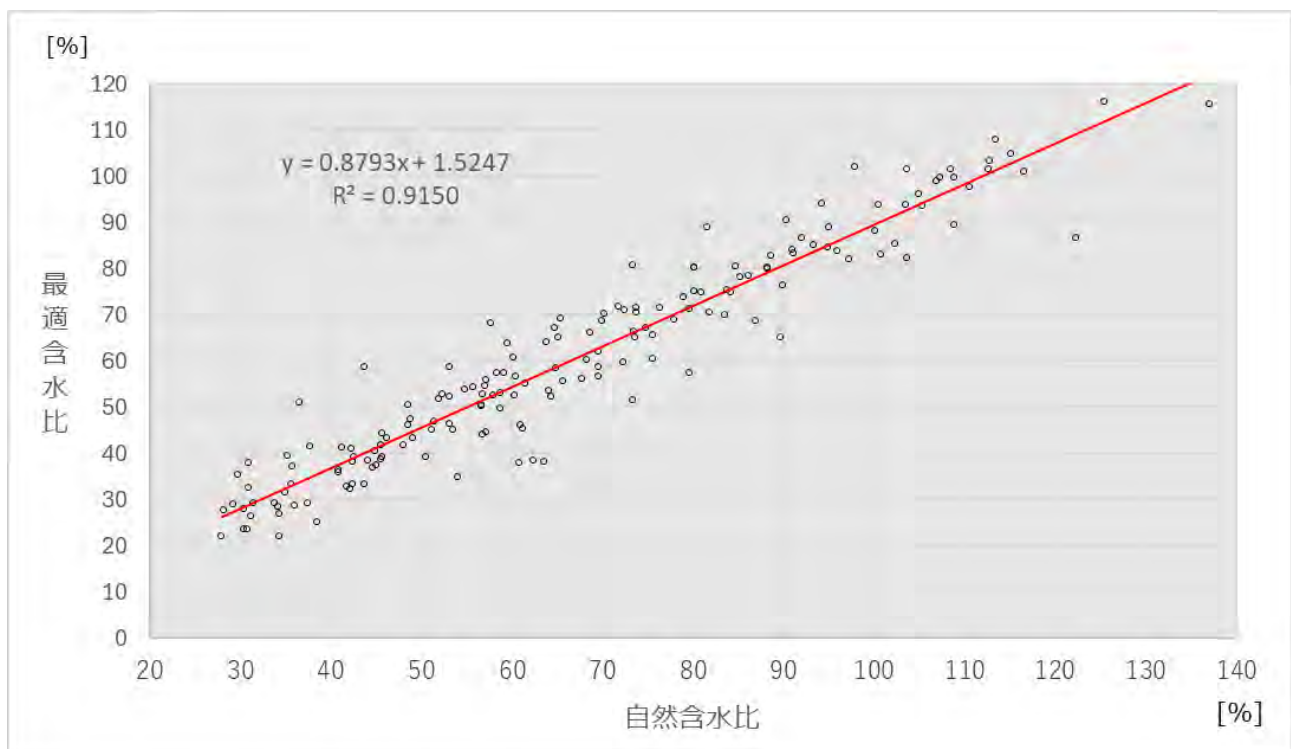
図－２ 自然含水比と最適含水比の関係（粘性土）
