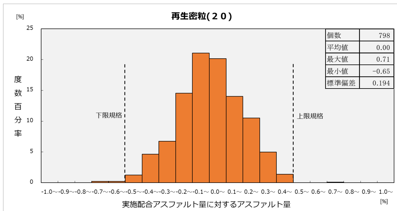
図3－（1）アスファルト量ヒストグラム
