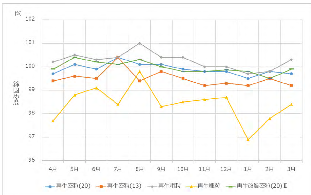
図－8 締固め度の月別平均変動
