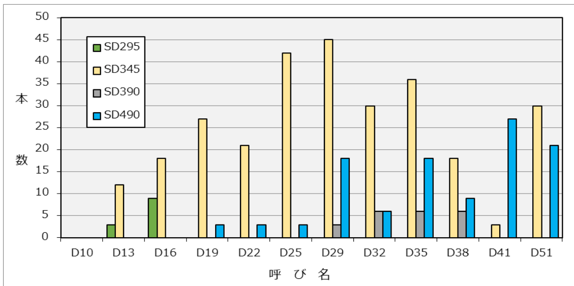
図－３ 機械式継手の呼び名別試験本数
