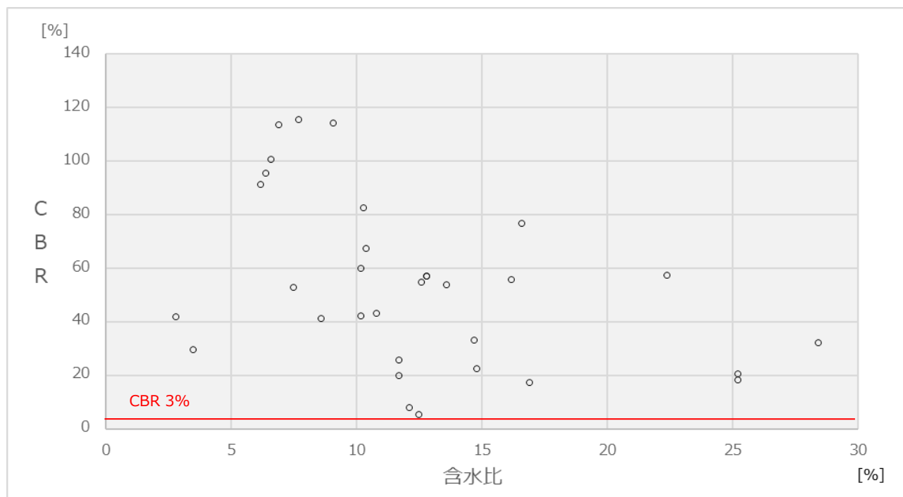
図－6 含水比とCBRの関係(れき質土)
