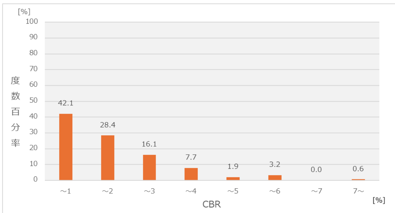
図－１１ C B R の分布(火山灰質細粒度)
