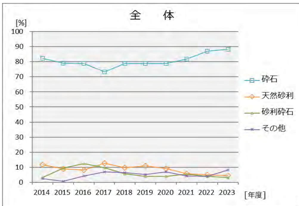
図2-1(1) 年度別粗骨材使用割合
