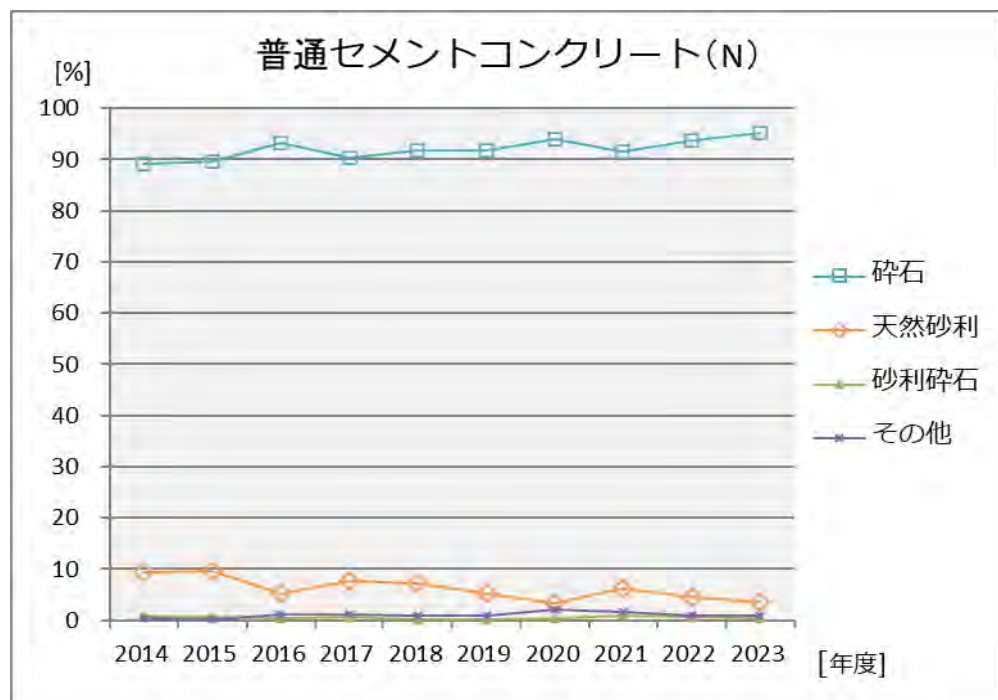
図2-1(2) 年度別粗骨材使用割合
