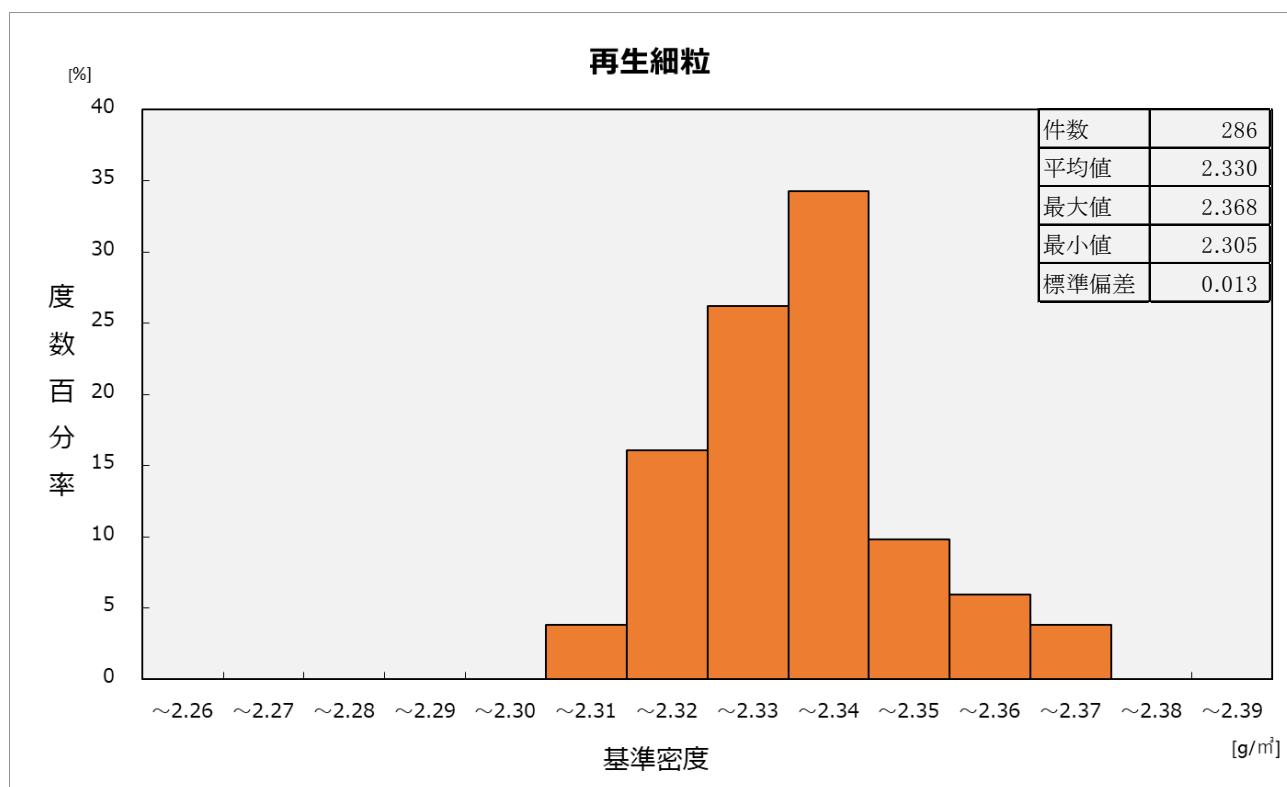
図ー 5 （ 4 ） 基準密度ヒストグラム
