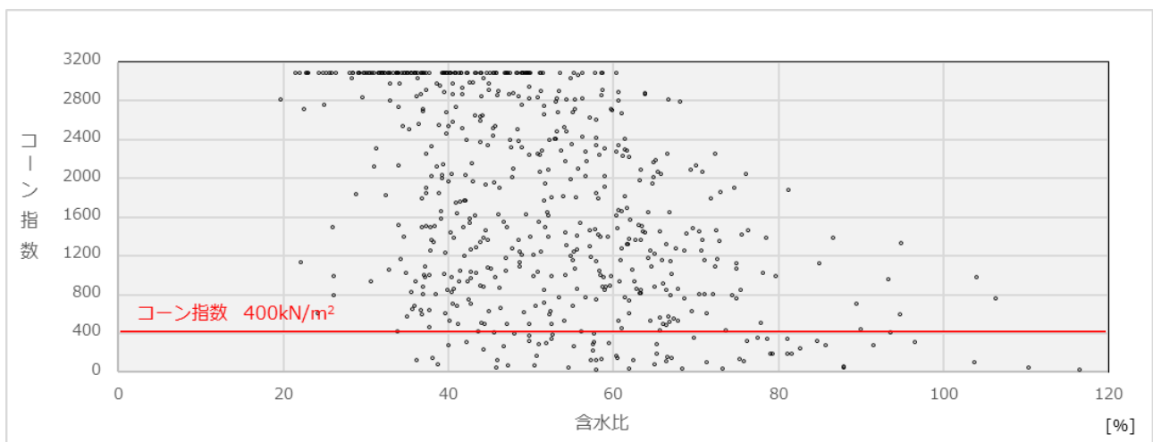
図－２０ コーン指数と含水比の関係(粘性土)
