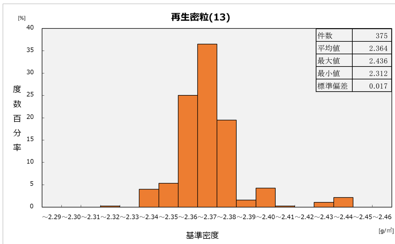
図ー 5 （ 2 ） 基準密度ヒストグラム
