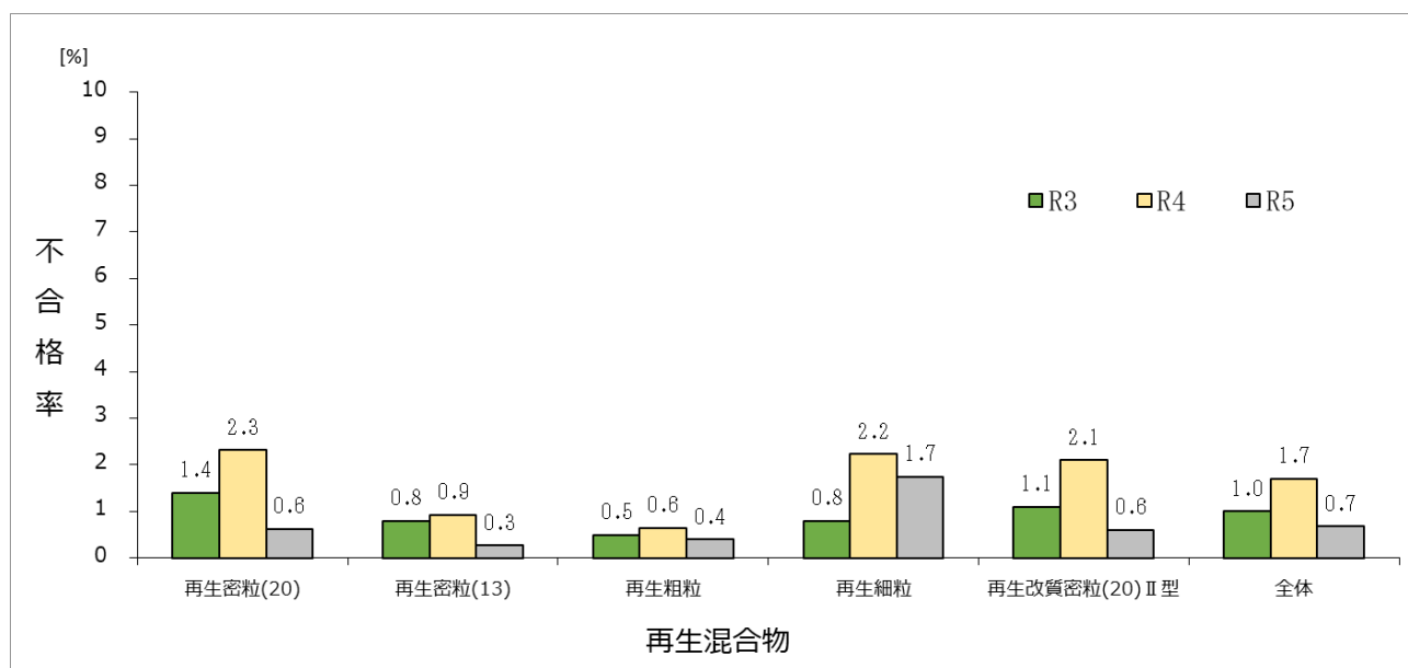
図－4 年度別アスファルト量の不合格率
