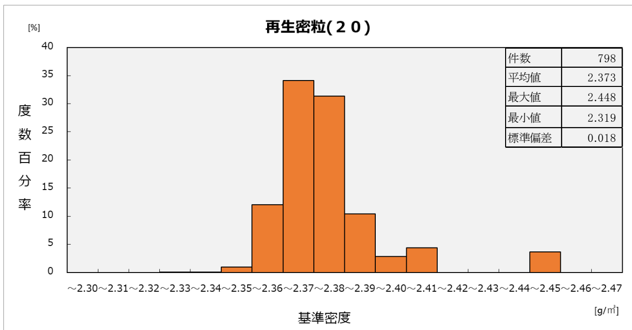
図－5（1） 基準密度ヒストグラム
