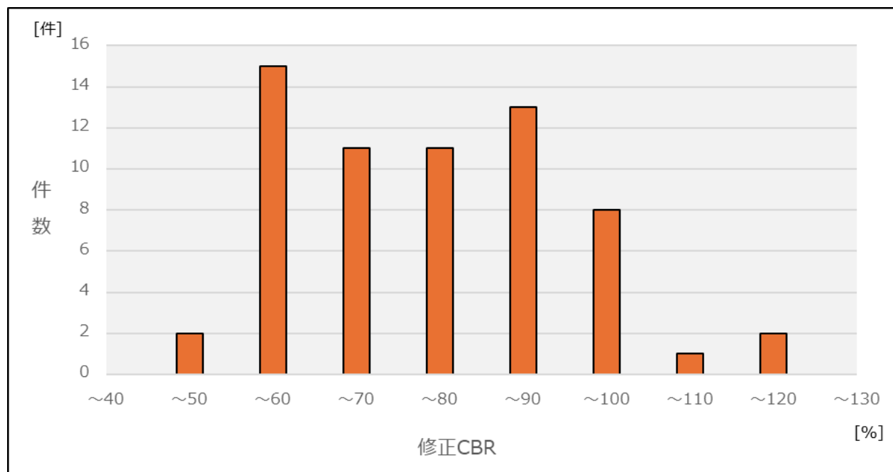
図-4 修正CBRの分布(C-40)
