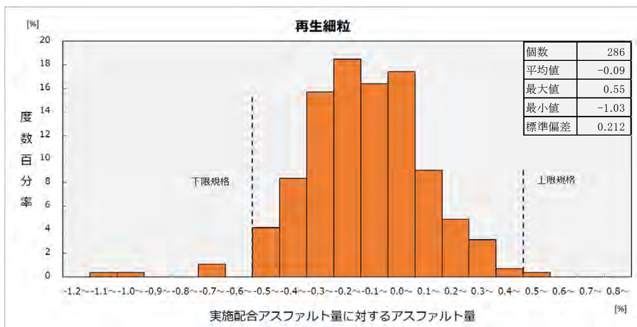
図 3 - (4) アスファルト量ヒストグラム
