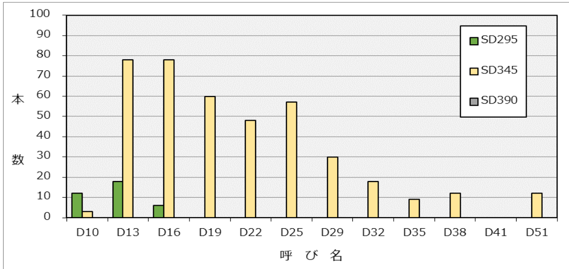
図－１ 素材の呼び名別試験本数
