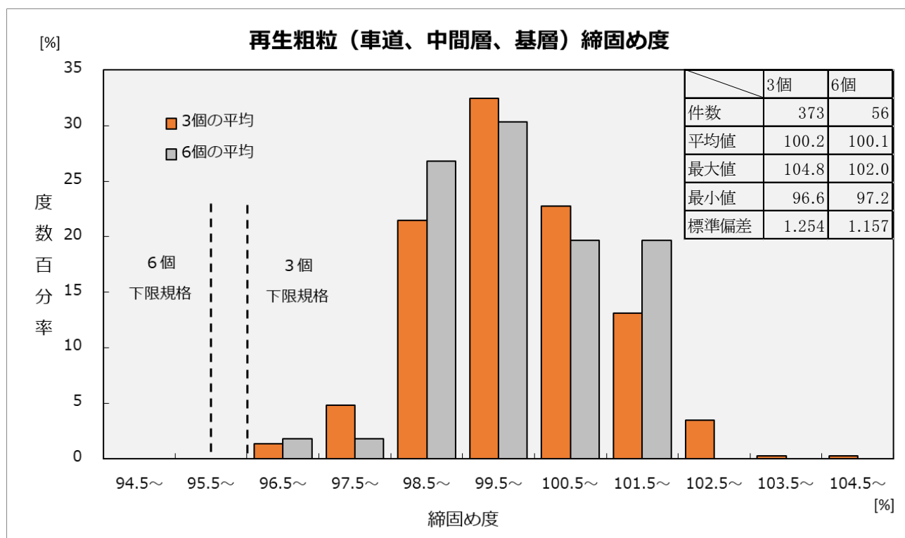
図ー 6 (3) 締固め度ヒストグラム
