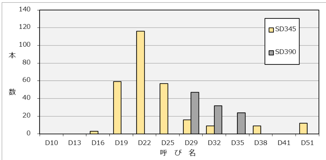
図－２ 圧接材の呼び名別試験本数
