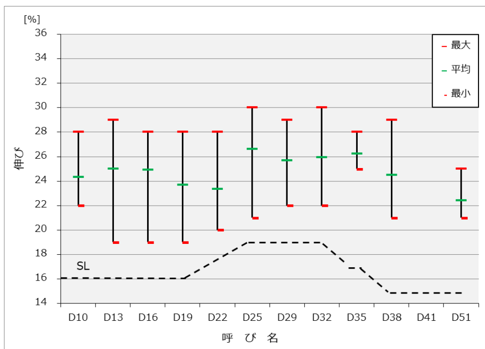
図－7 破断伸びの範囲 (SD345)
