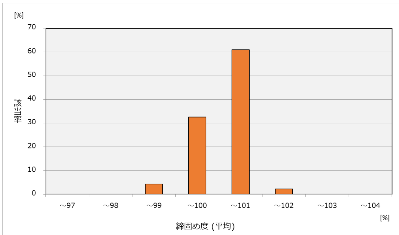
図－ 9 （ 3 ） 締固め度 再生改質Ⅱ型粗粒
