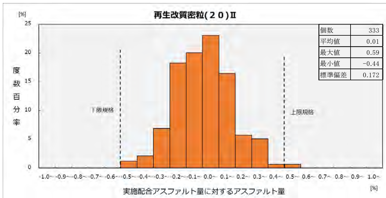
図3－(5) アスファルト量ヒストグラム
